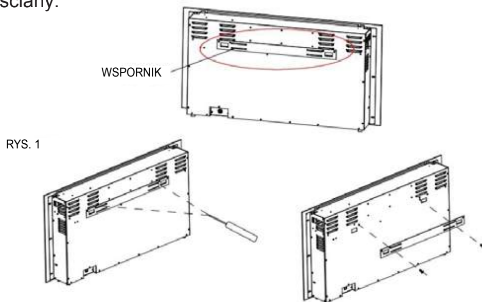
Ilustracja przedstawiająca wspornik ścienny dla modeli AV-INS32-39PRO
